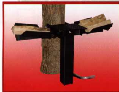
Tisch für nur 50 cm Spalthöhe mit seitlichen Verbreiterungen und Pedalsteuerung für das Ausrichten des Spaltholzes! Artikelnr. 845.034.K
